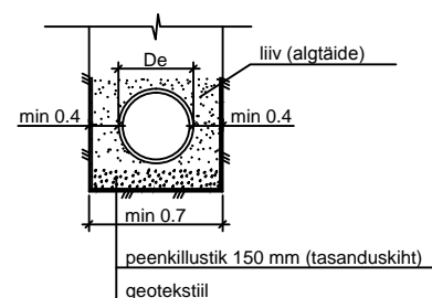
Toru alus geotekstiiliga
