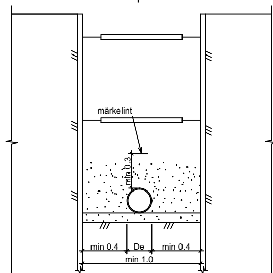
Kaeviku ristlõige Tüüp nr 1
